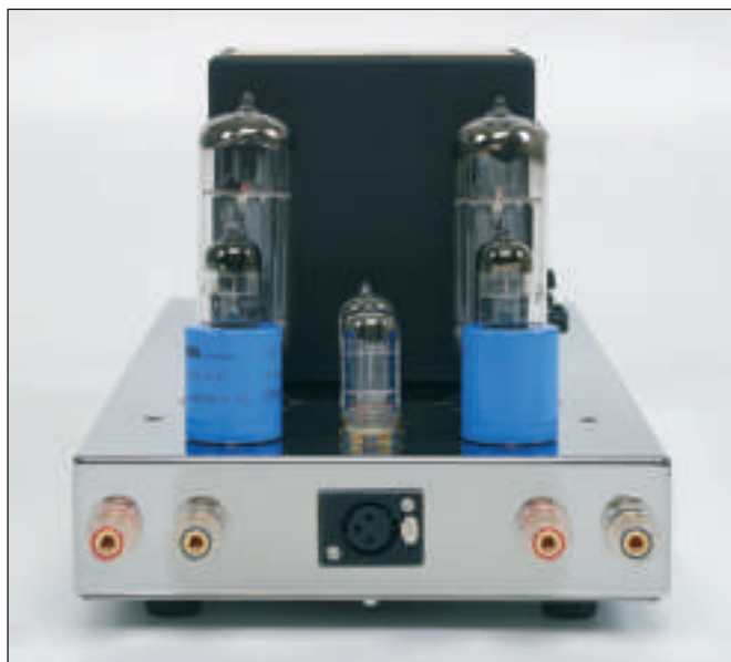
Il pannello posteriore del JA-50 è piuttosto semplice. Un ingresso bilanciato e uscita per diffusori sdoppiata. Le valvole finali (le più alte) sono delle KT90
