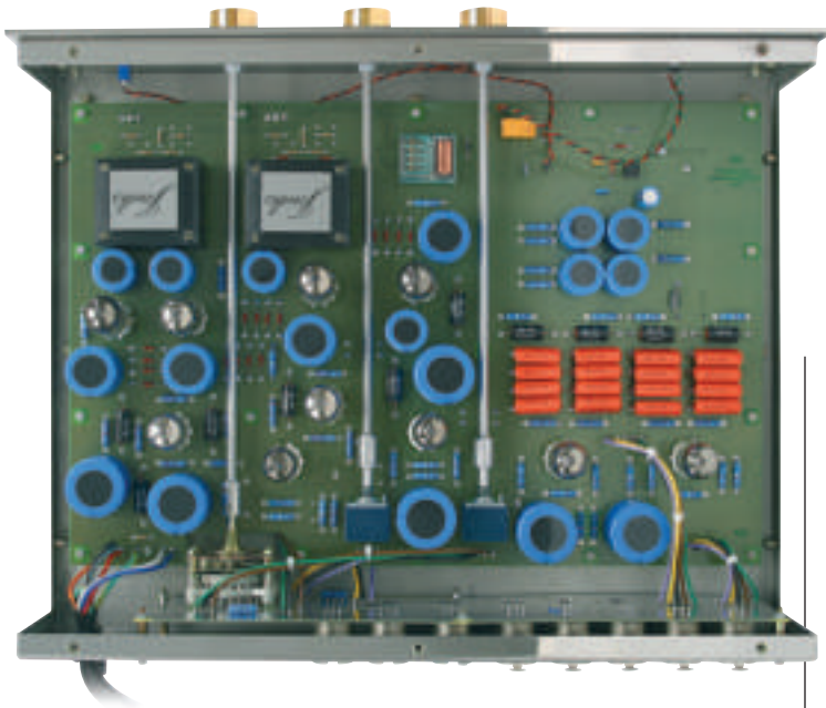
L'interno del preamplificatore JPS-8 denota una costruzione di livello assoluto, e eccezionalmente ordinata. Nulla è lasciato al caso e tutti i componenti sono selezionati.
